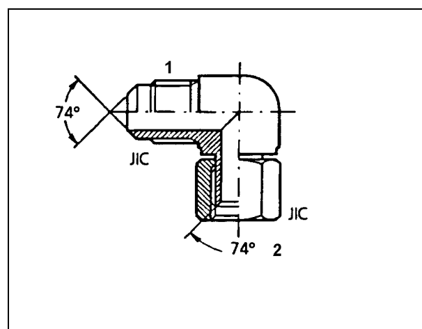
A30JM90-30JF 1"7/8-12 1"7/8-12
