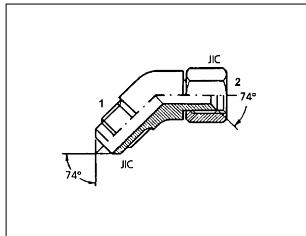
A30JM45-30JF 1"7/8-12 1"7/8-12
